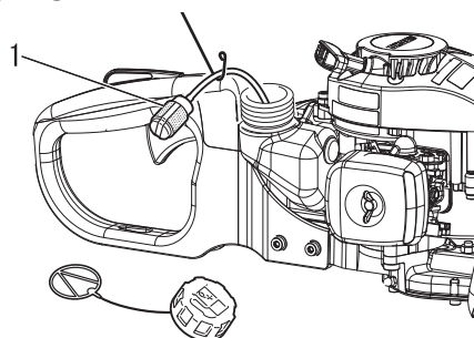
1. Kraftstofffilter
