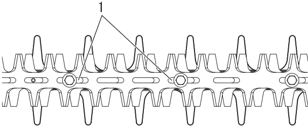
1. Schraubenschlitze
